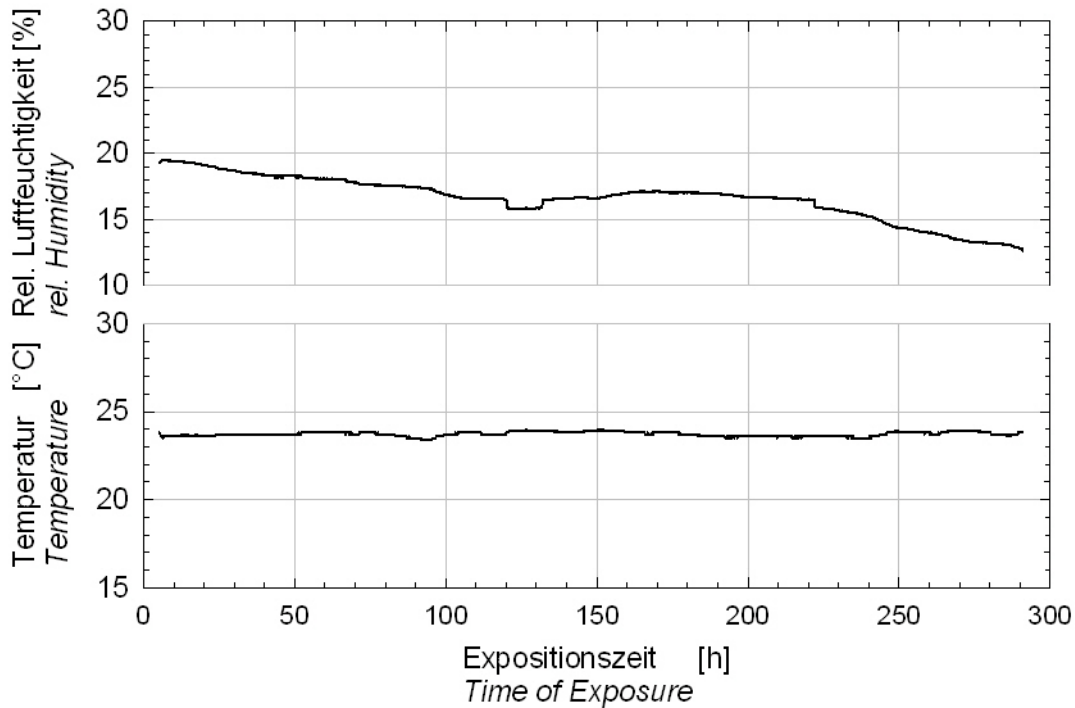
Abbildung 6-3: Temperatur und relative Luftfeuchtigkeit während der Expositionen / Temperature and relative humidity during the exposures
