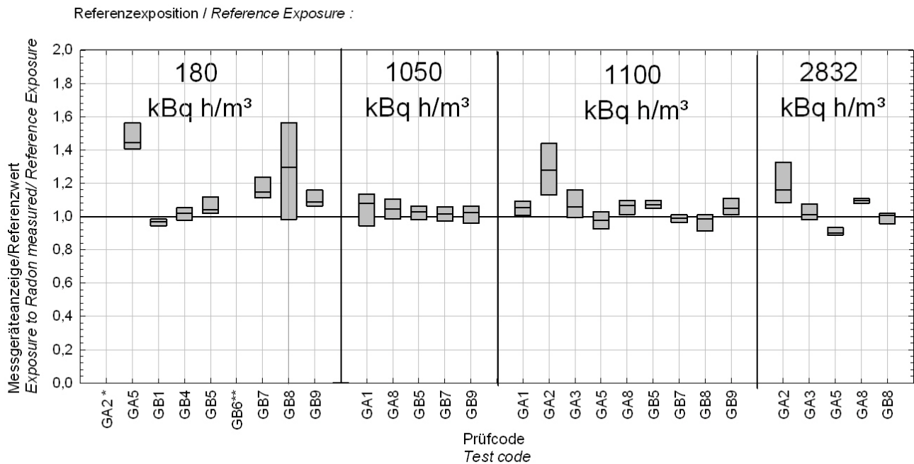
Abbildung 4-5: Relative Messabweichung der Messgeräte mit Elektret der Expositionsgruppen 1 bis 4/ Relative error of the instruments using electrets of the exposure groups 1 to 4
