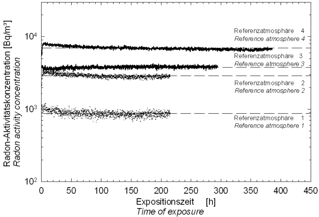
Abbildung 6-2: Zeitlicher Verlauf der Radon-Aktivitätskonzentrationen der Referenzatmosphären / Radon activity concentrations of the reference atmospheres versus time of exposure
