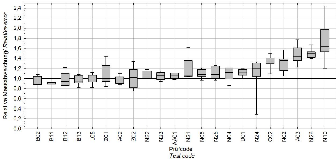
Abbildung 4-1: Relative Messabweichung der Messgeräte mit Kernspurdetektoren der Expositionsgruppe 1 / Figure 4-1: Relative error of the instruments using nuclear track detectors of exposure group 1
