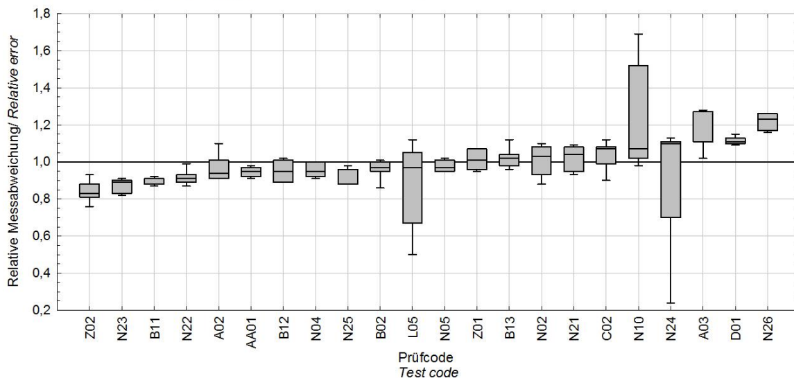
Abbildung 4-4: Relative Messabweichung der Messgeräte mit Kernspurdetektoren der Expositionsgruppe 4 / Figure 4-4: Relative error of the instruments using nuclear track detectors of exposure group 4
