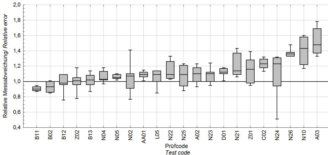
Abbildung 4-2: Relative Messabweichung der Messgeräte mit Kernspurdetektoren der Expositionsgruppe 2 / Figure 4-2: Relative error of the instruments using nuclear track detectors of exposure group 2
