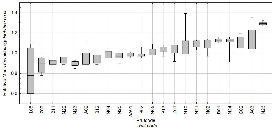
Abbildung 4-3: Relative Messabweichung der Messgeräte mit Kernspurdetektoren der Expositionsgruppe 3 / Figure 4-3: Relative error of the instruments using nuclear track detectors of exposure group 3
