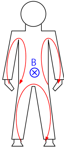
Abbildung 6.3: Ausgeprägte „Schleifenstrukturen“ die bei magnetischer Ganzkörperexposition von vorne bzw. hinten zu großen induzierten elektrischen Feldstärken in der Haut der Finger- und/oder Zehenspitzen führen können.
