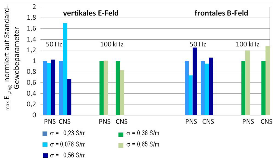
Abbildung 4.25: Einfluss der Muskelleitfähigkeit auf die induzierten Feldstärken in CNS- und PNS-Geweben. Körpermodell Roberta. Maximale induzierte, über 2 \times 2 \times 2 \text{ mm}^3 gemittelte elektrische Feldstärke, normiert auf die Ergebnisse mit den Standard-Leitfähigkeitswerten
