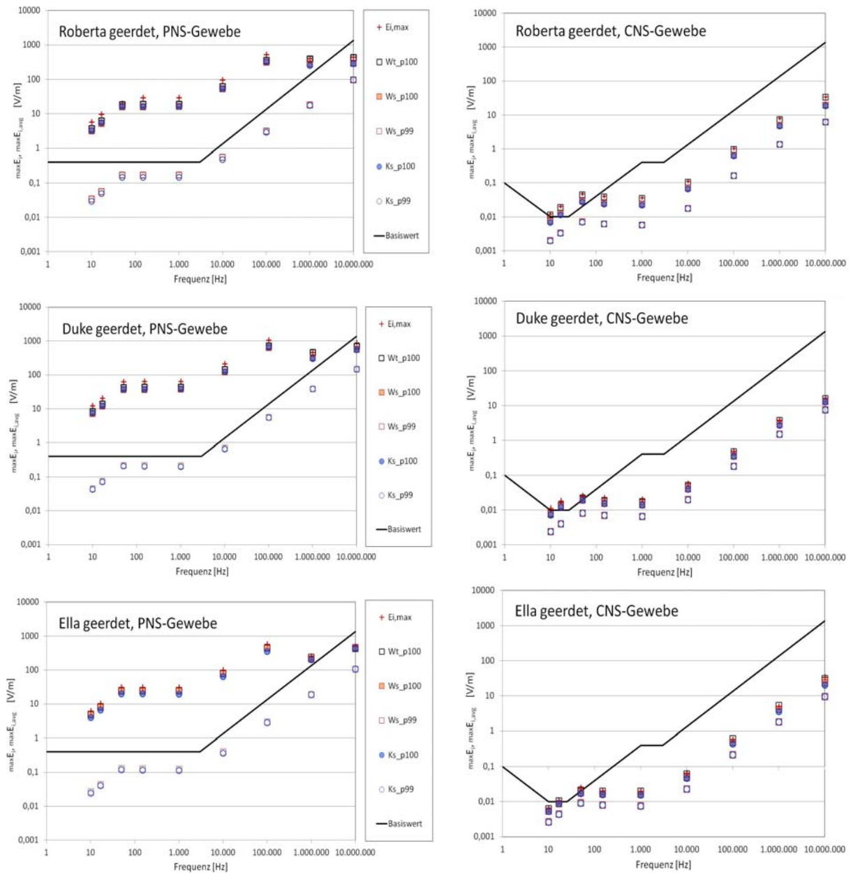
Abbildung 4.19: Vergleich der mit den unterschiedlichen Körpermodellen und unterschiedlichen Mittelungsmethoden erhaltenen Berechnungsergebnisse mit den jeweiligen Basiswerten (links PNS-Gewebe, rechts: CNS-Gewebe). Alle Körpermodelle sind geerdet. Vertikale, homogene elektrische Feldstärke entsprechend dem Referenzwert für die Allgemeinbevölkerung gemäß ICNIRP 2010.
