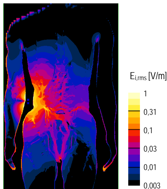
Abbildung 5.21: Verteilung der ungemittelten induzierten elektrischen Feldstärke im betrachteten Szenario in einer Vertikalebene durch das Maximum.
