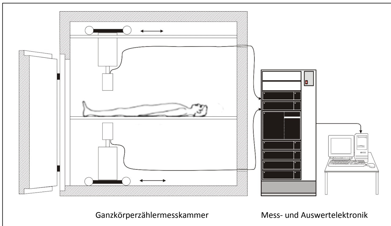
Abbildung 2: Schematischer Aufbau der Ganzkörpermessanlage
