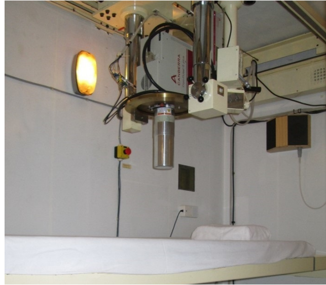
Abbildung 3a: Kalibrierphantom (70-kg-Konfiguration). Abbildung 3b: Oberer Detektor mit elektrischer Kühlung.
