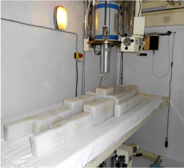
Abbildung 3a: Kalibrierphantom (70-kg-Konfiguration). Abbildung 3b: Oberer Detektor mit elektrischer Kühlung.
