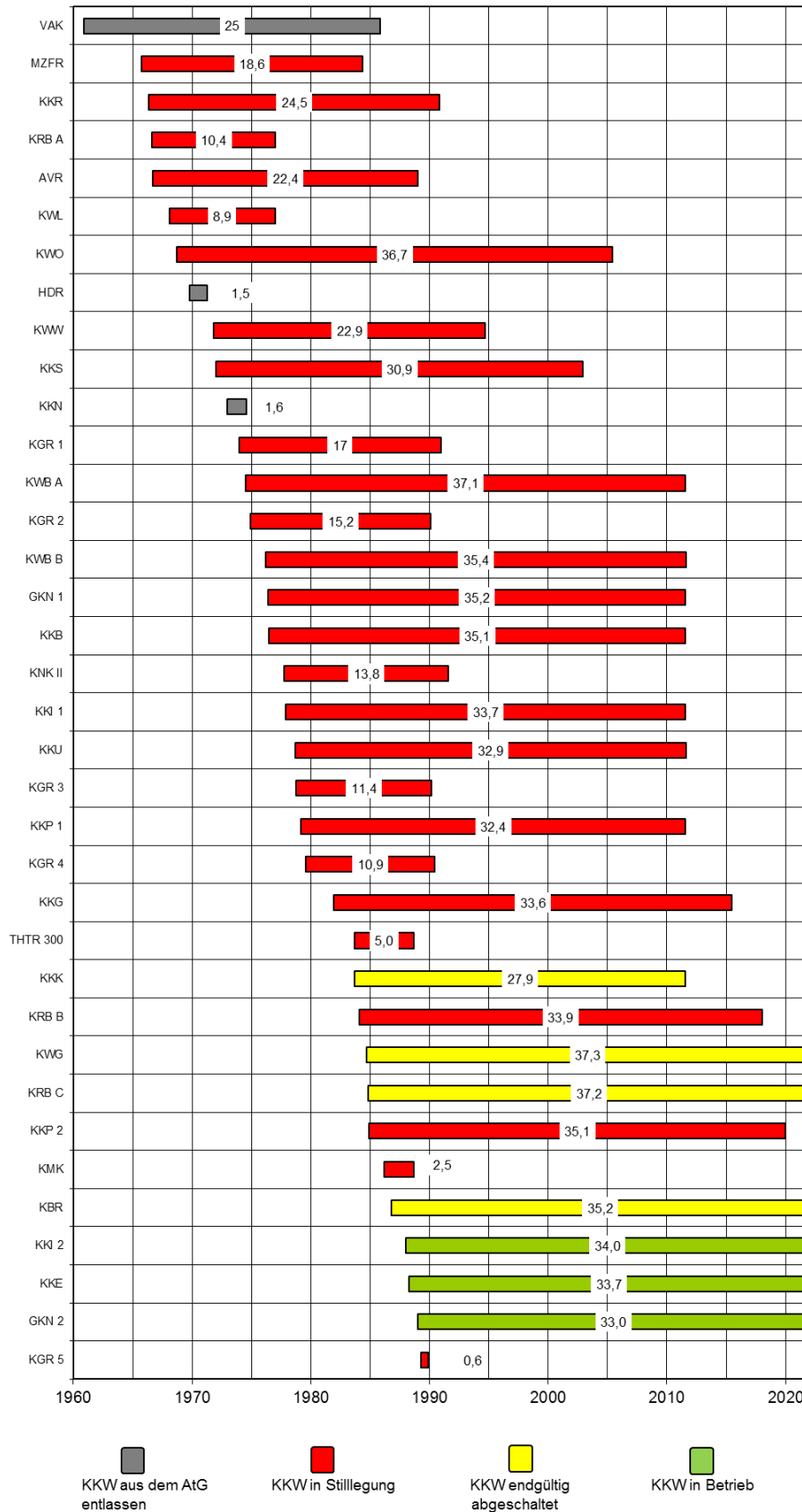
Abb. 2: Betriebszeiten der Kernkraftwerke in Deutschland in Jahren seit Erstkritikalität Stand 31.12.2021 24:00 Uhr MEZ
