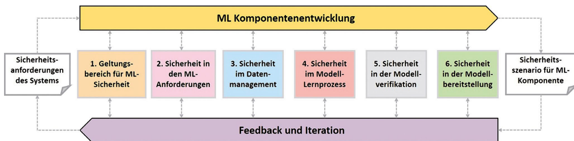
Abb. 4.1 Übersicht über den AMLAS-Prozess /HAW 21/, entnommen aus /WU 21/.
