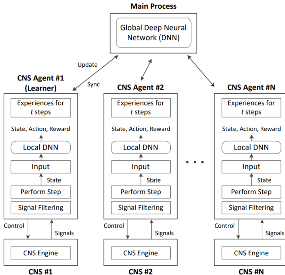
Abb. 5.2 Lernstruktur mehrerer Agenten. /HIN 98/
