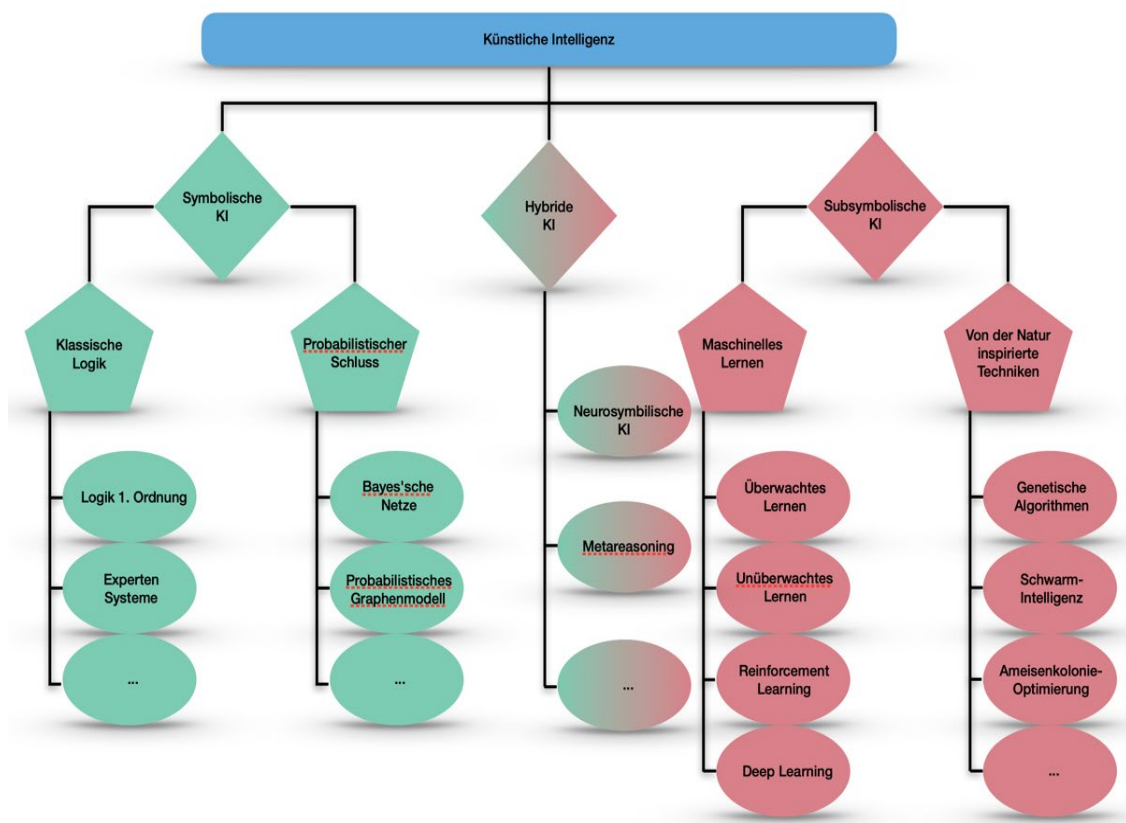
Abb. 2.1 Klassifikation von KI-Methoden (eigene Darstellung) /IEC 23/.
