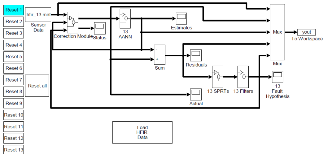
Abb. 5.1 Beispielsrealisierung des AANN/SPRT-Überwachungssystems
