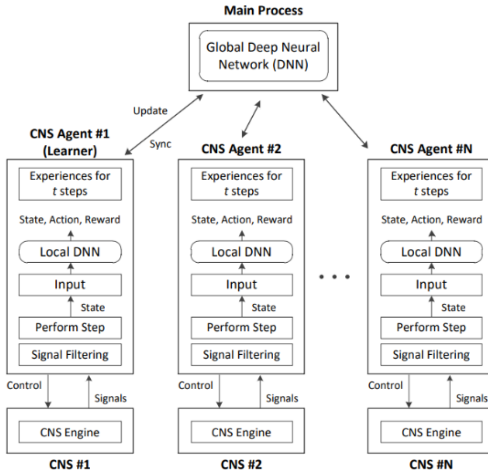
Abb. 2.7 Beispielhafte Lernstruktur multipler Agenten. /PAR 22/
