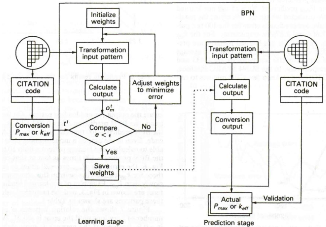
Abb. 5.3 Prozedurale Darstellung des Lern- und Vorhersagealgorithmus. /KIM 93/
