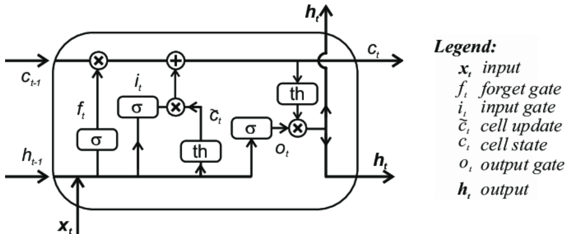
Abb. 2.6 Beispielhafte Darstellung einer LSTM-Zelle. /HRN 19/
