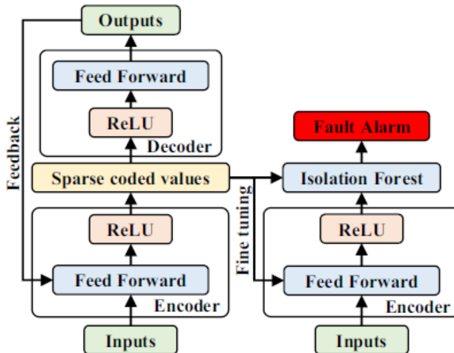
Abb. 5.4 Strukturdiagramm des Algorithmus zur Anomalieerkennung. /LI 22a/
