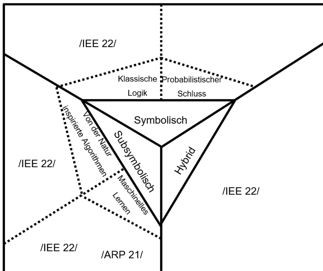
Abb. 3.1 Einordnung von KI-basierten Anwendungen nach /IEC 23/.
