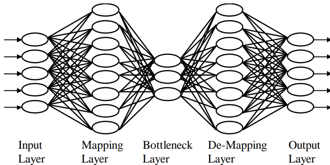
Abb. 2.5 Beispiel eines AANN. /HIN 98/
